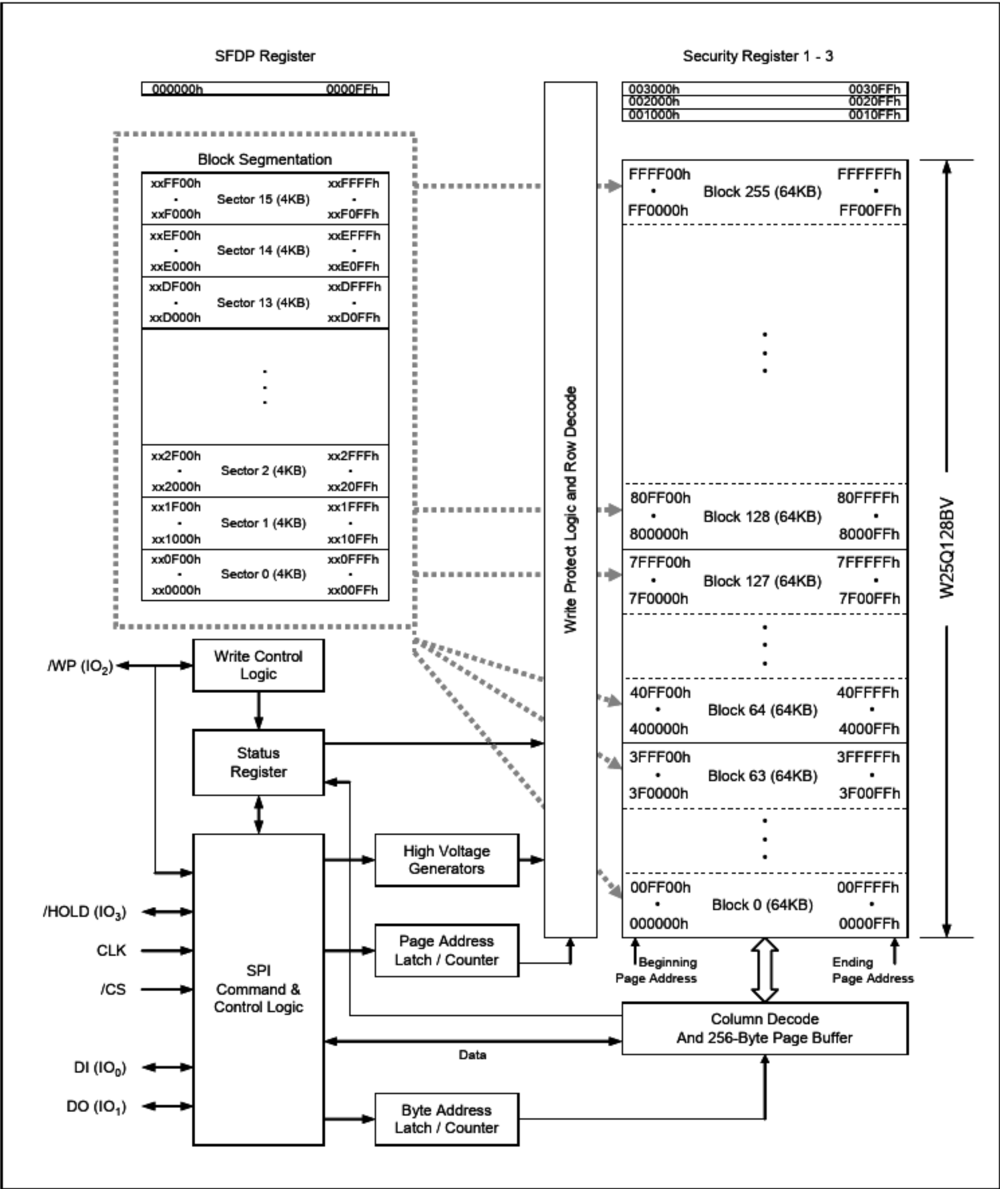
图2. W25Q128BV串行闪存框图
