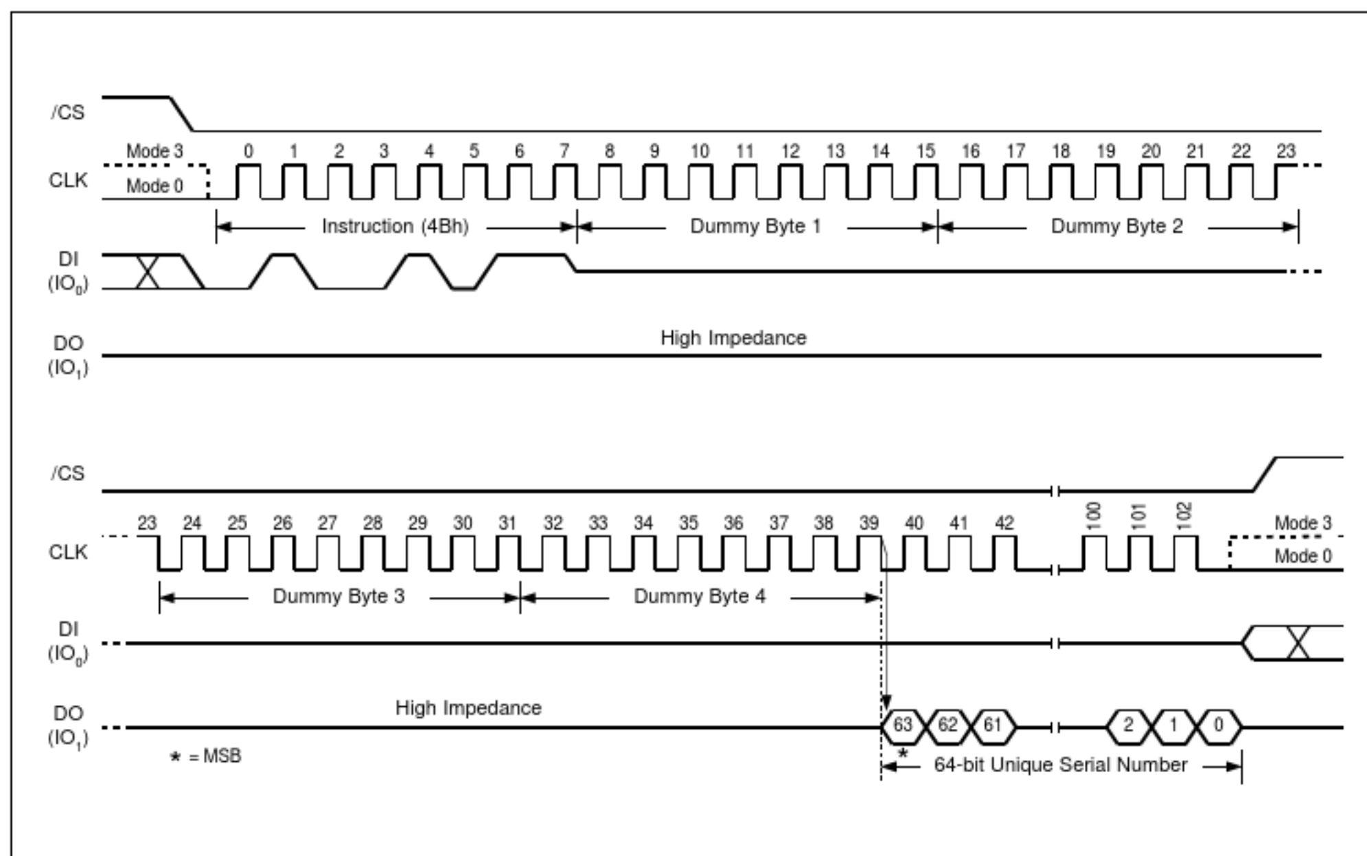
图32.读唯一的ID号指令序列
