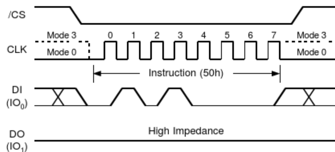
图5.写使能挥发性状态寄存器指令序列图
