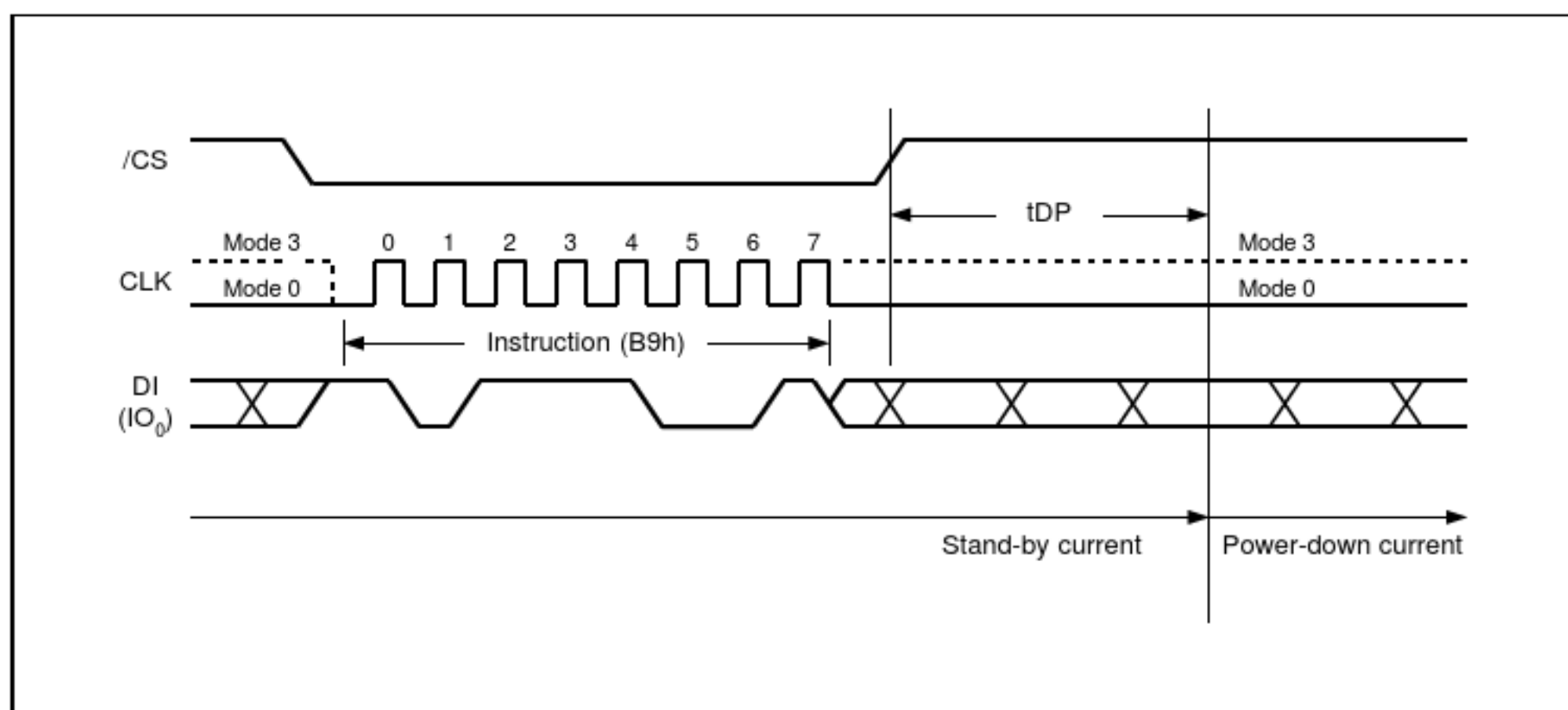
图27. Deep Power-down 指令序列图
