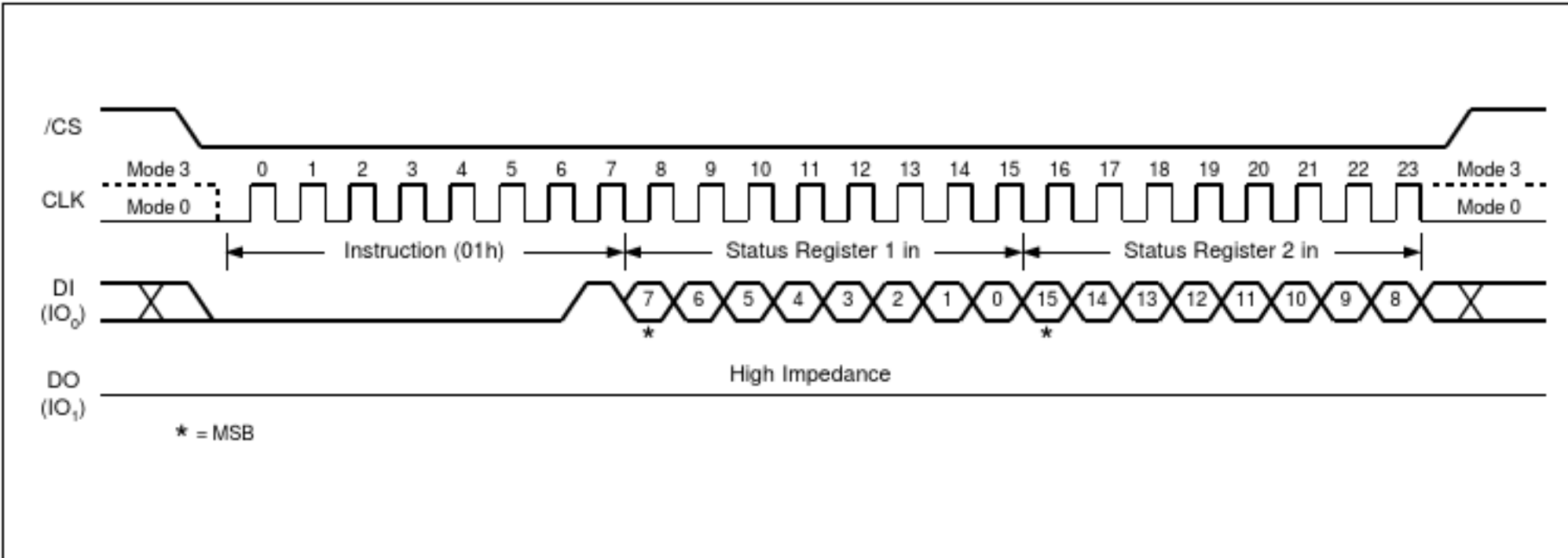
图8.写状态寄存器指令序列图
