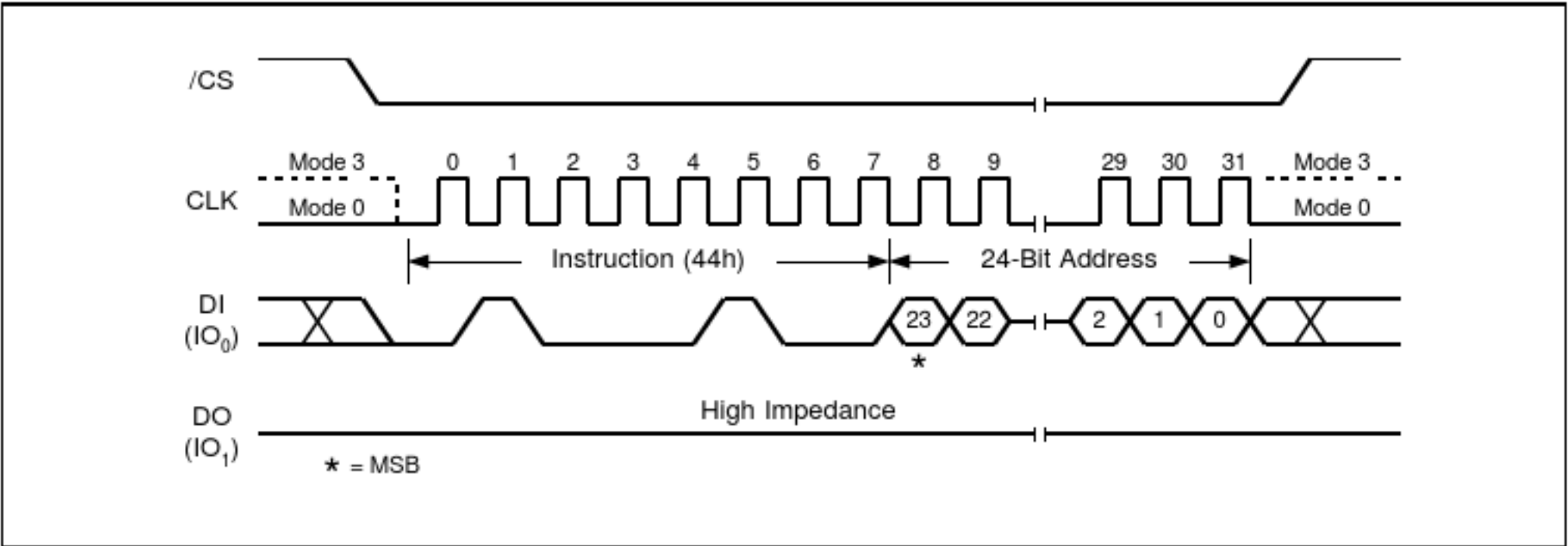
图35.擦除安全寄存器指令序列
