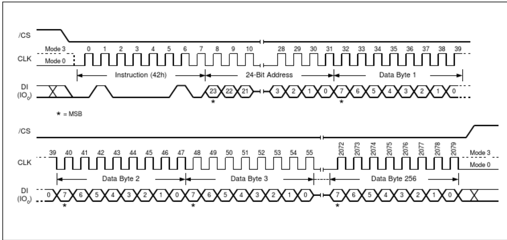
图36.编程安全寄存器指令序列
