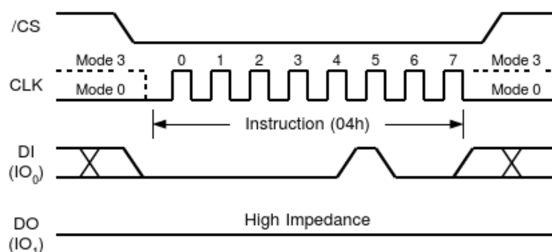
图6.写禁止指令序列图
