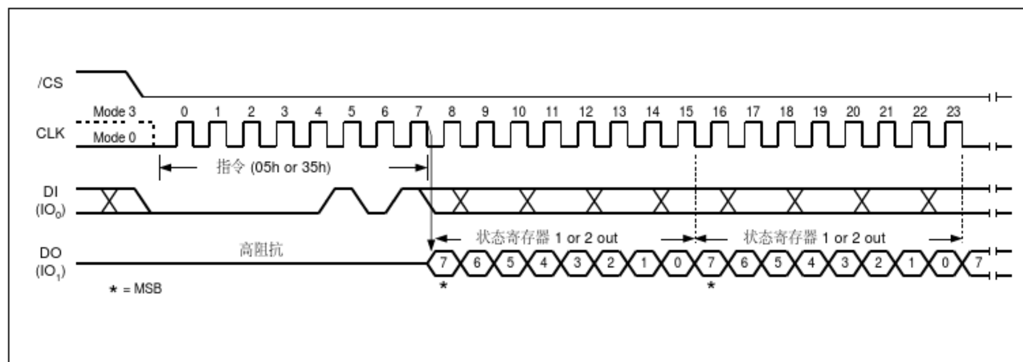
图7.读状态寄存器指令序列图
