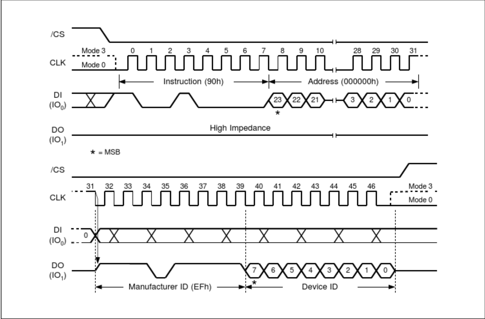
图29.读制造商/设备ID图
