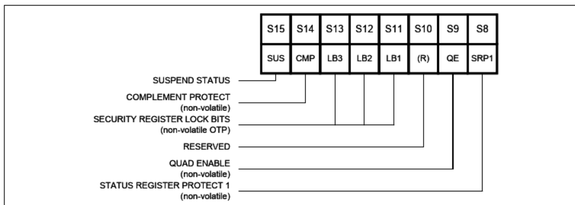
图3b。状态寄存器-2
