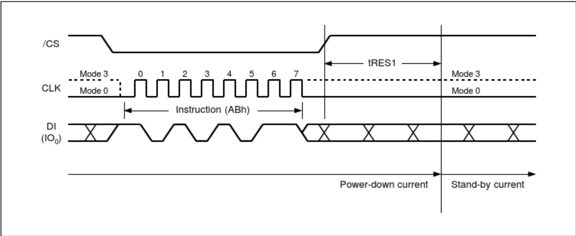
图28A. 释放掉电指令序列
