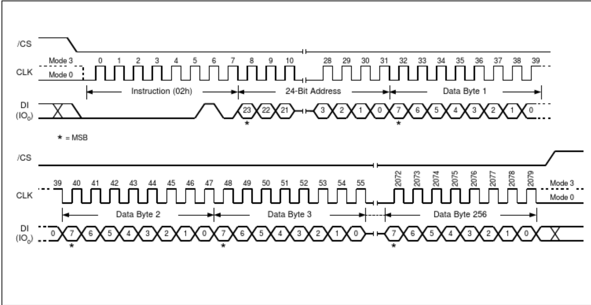
图19.页面编程指令序列图
