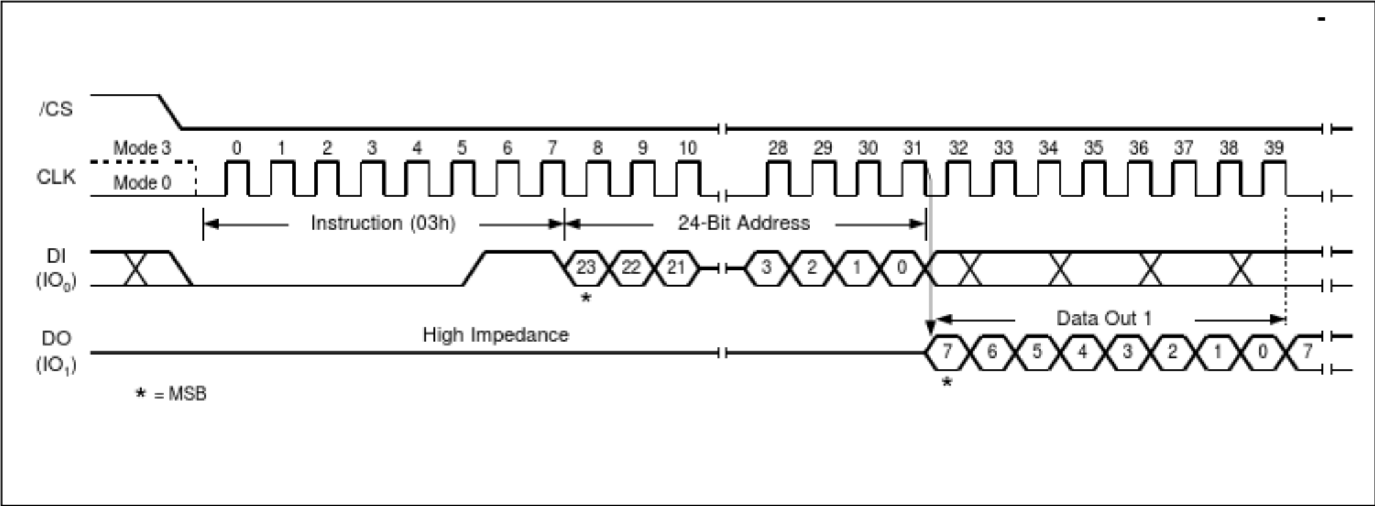
图9.读取数据指令序列图
