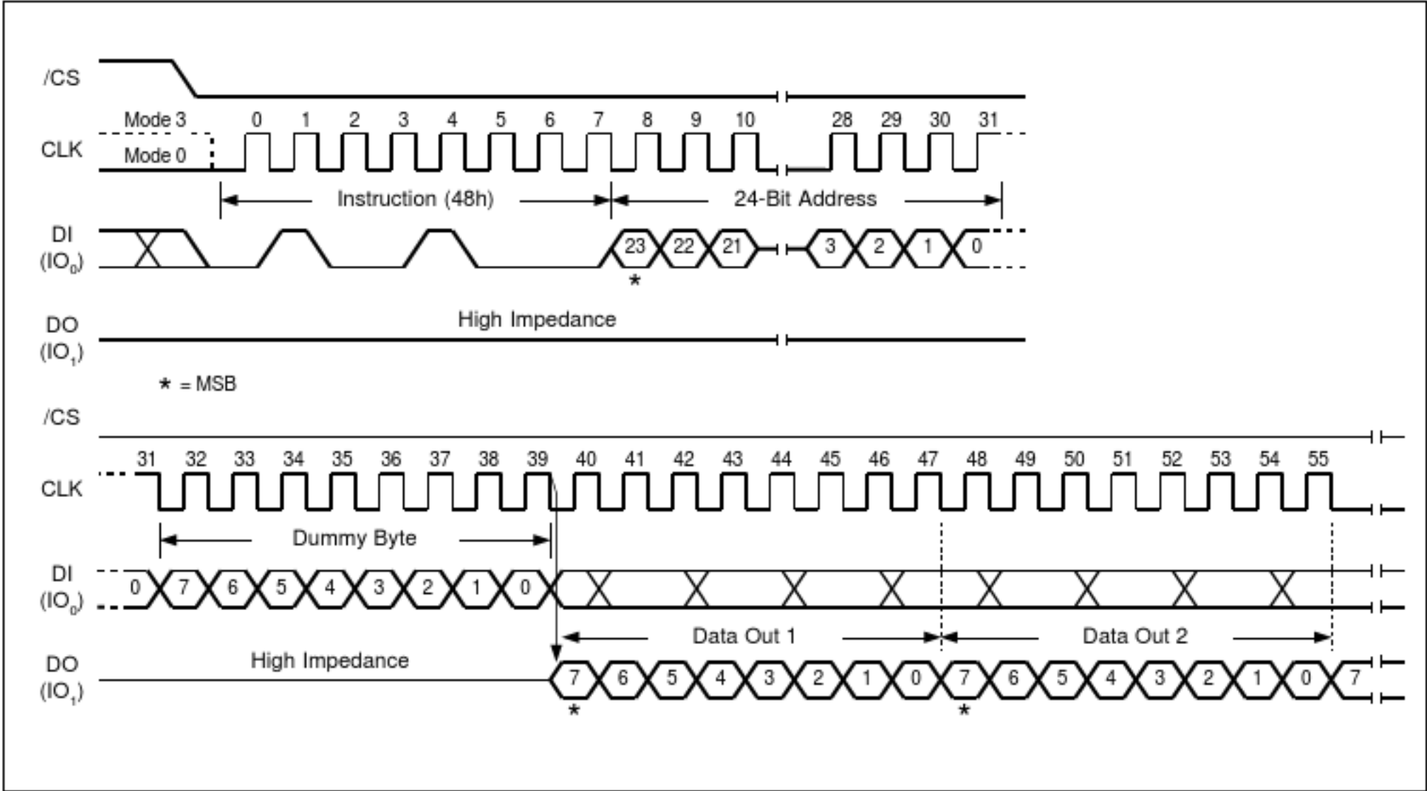
图37.读安全寄存器指令序列
