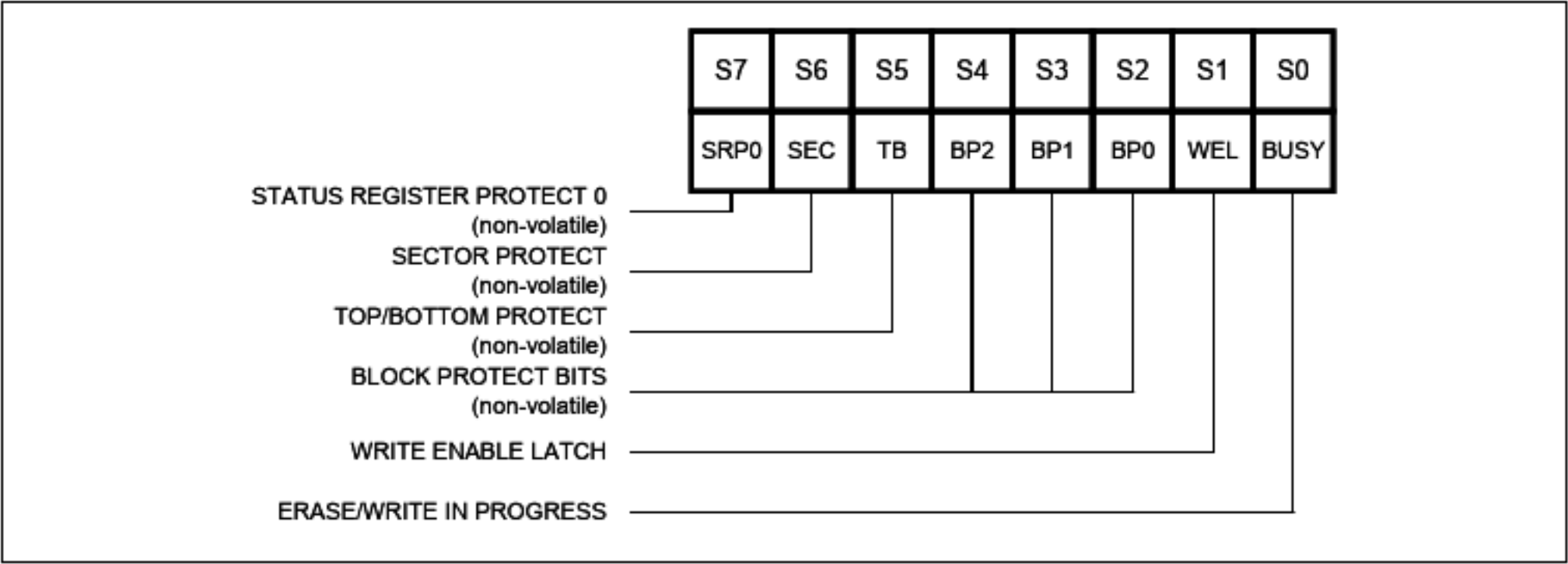
图3a。状态寄存器-1
