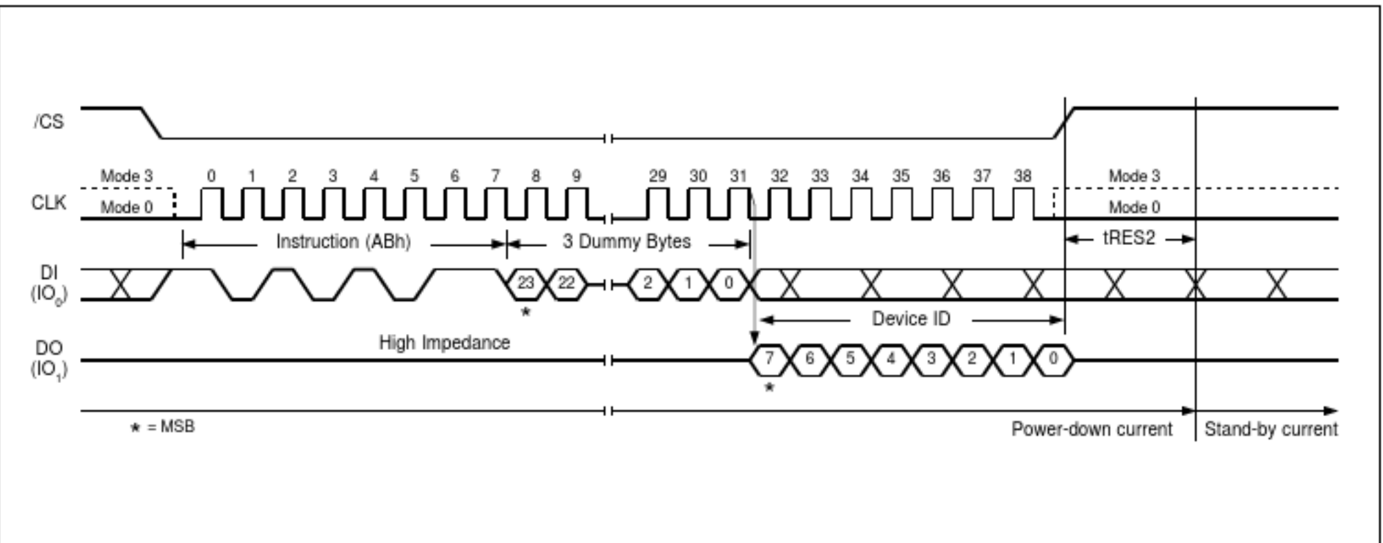
图28B. 释放掉电/设备ID指令序列图
