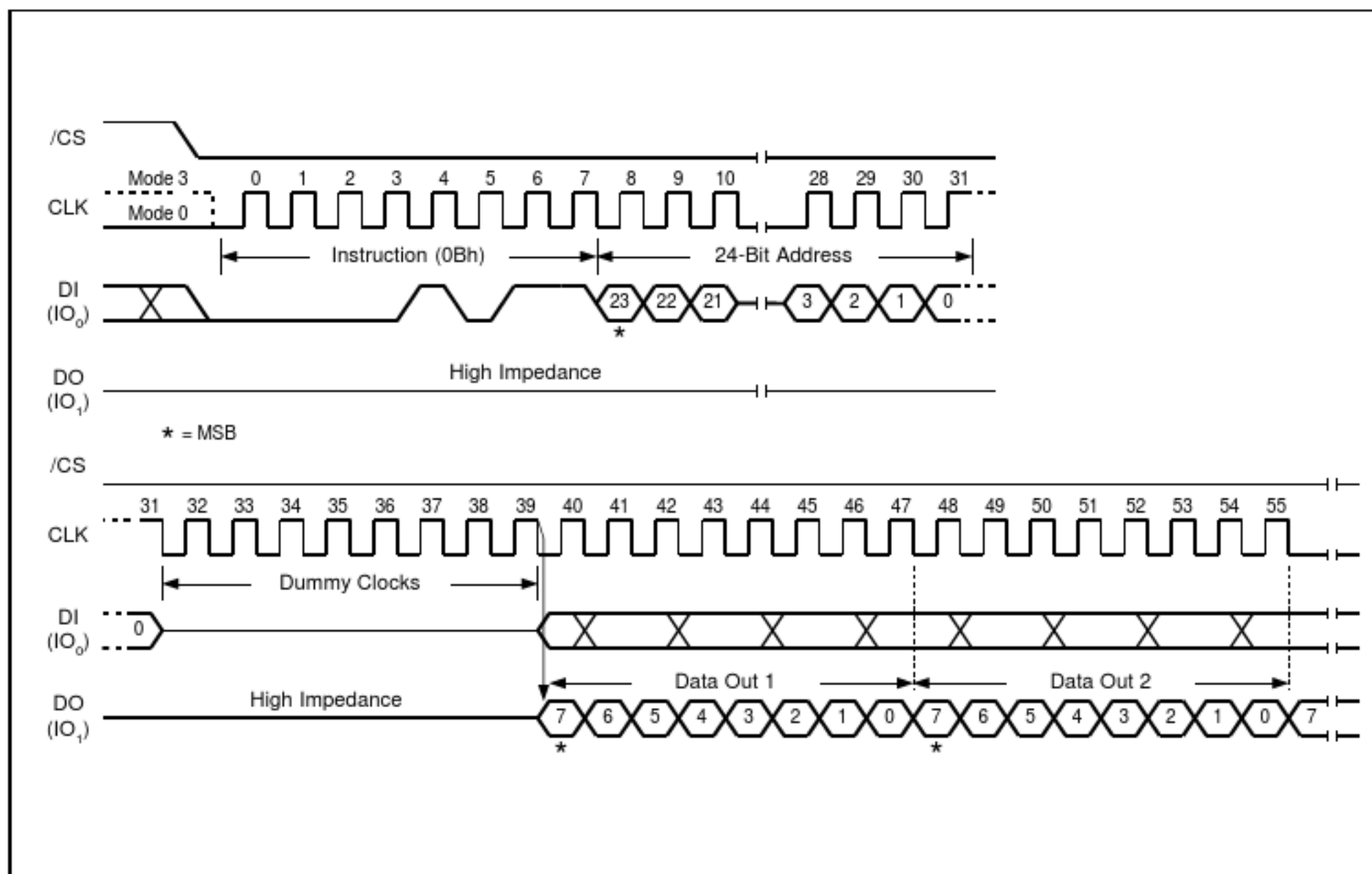
图10.快速读取指令序列图
