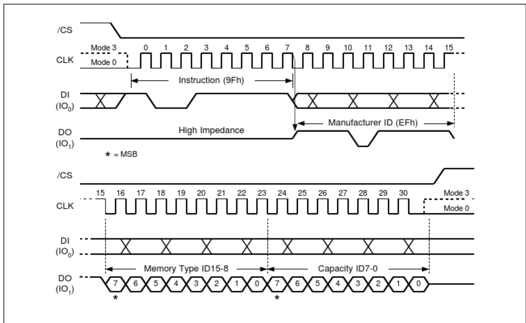
图33.读JEDEC的ID指令序列
