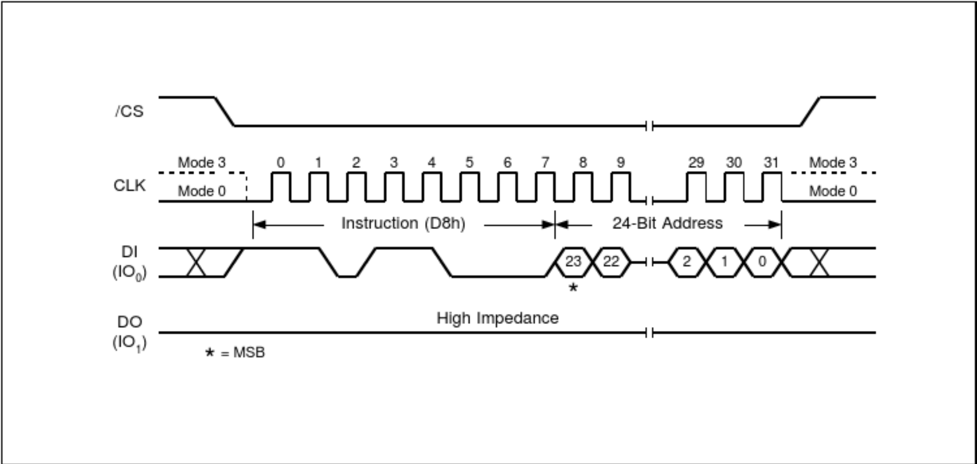
图23.64KB块擦除指令序列图
