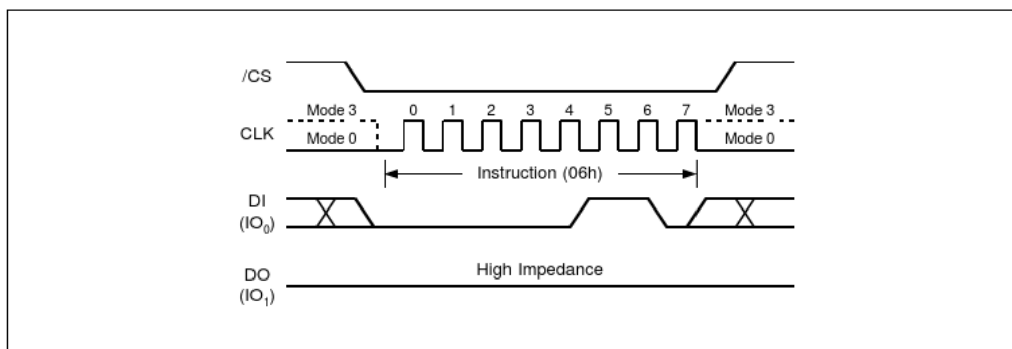
图4.写使能指令序列图
